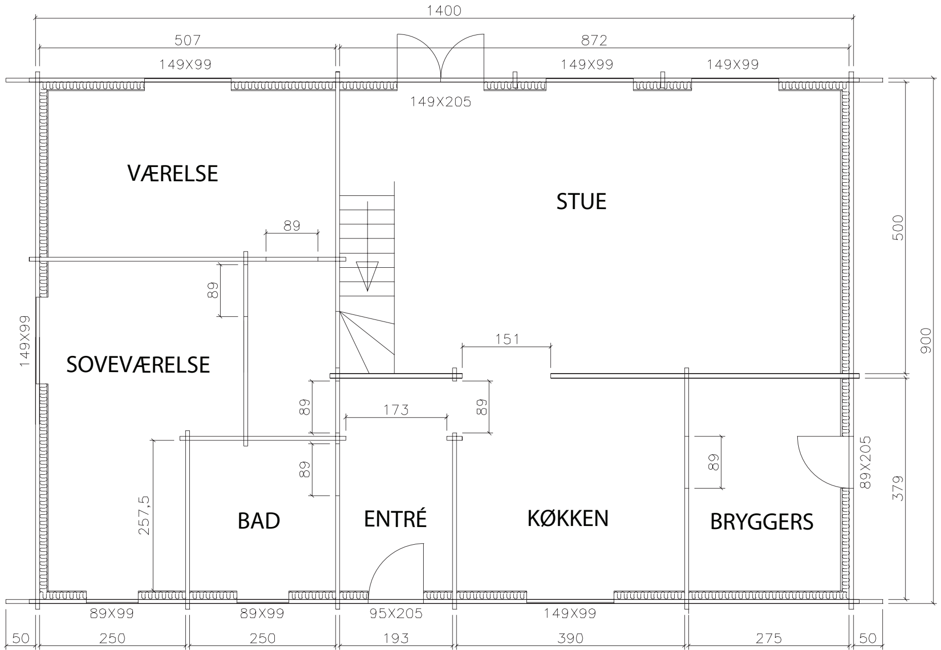
GRUNDPLAN
